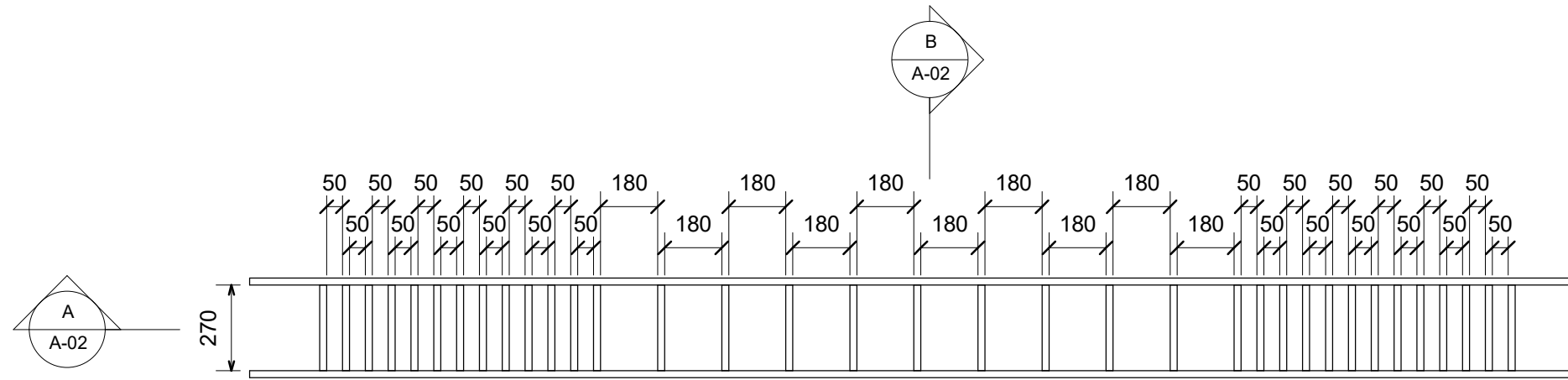
P PLAN 1 : 20
